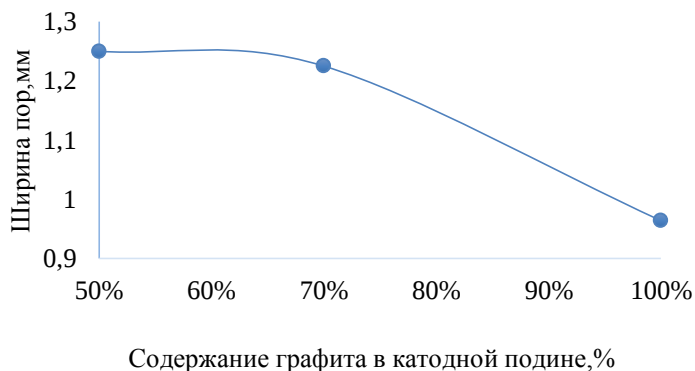
Рисунок 6 – Сравнительная диаграмма зависимость ширины трещин от содержания графита в образцах
