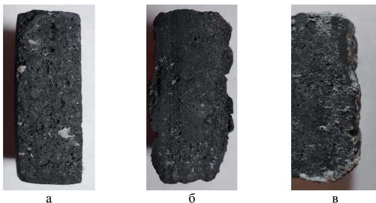
а – Образец с 50% содержанием графита; б – Образец с 70% содержанием; в – Образец с 100% содержанием графита.
