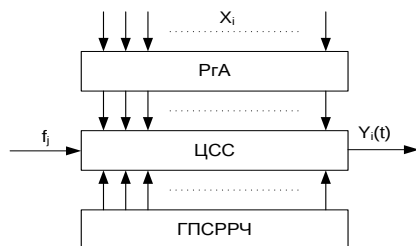
Рисунок 1 – Структурная схема преобразователя число – вероятностное отображения
