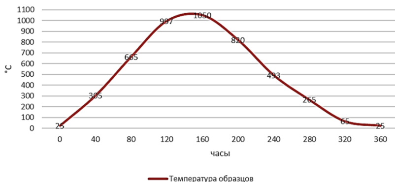
Рисунок 1 – Кривая обжига для испытываемых образцов
