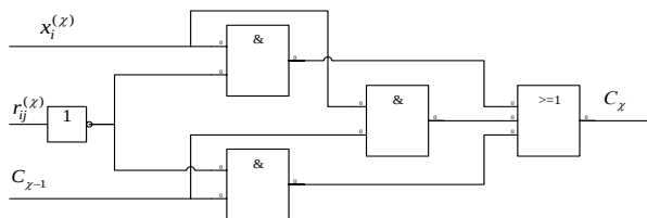
Рисунок 2 – Функциональная схема \chi -го разряда цифровой схемы сравнения, реализующая C_\chi
