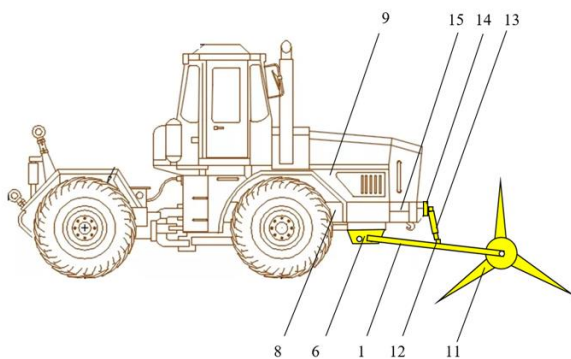
Рисунок 2 – Профильный вид колёсного полурамного трактора с установленным фронтальным прокалывателем-щелерезом
