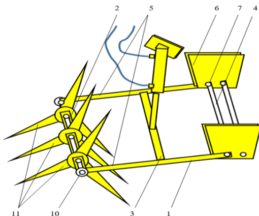
Рисунок 1 – Принципиальная схема фронтального прокалывателя-щелереза
