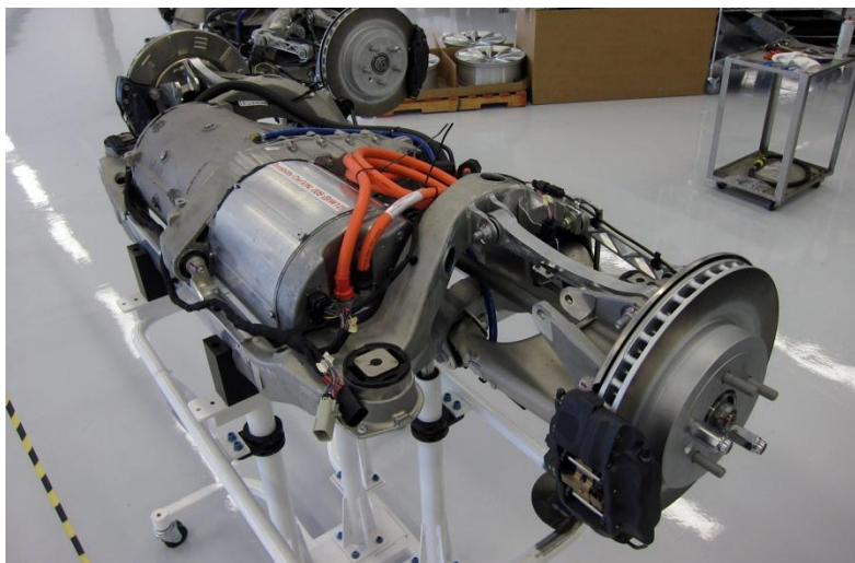
Рисунок 1 – Двигатель Tesla Model S
