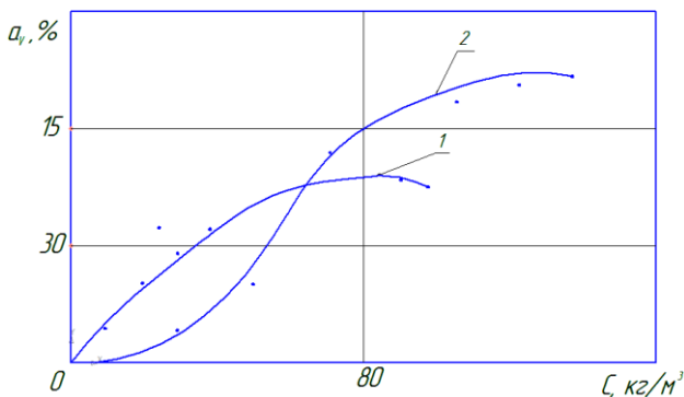
Рисунок 1 – Влияние содержания частиц С в электролите на включение в покрытие a_v электрокорунда белого марок 1– М7; 2 –М14
