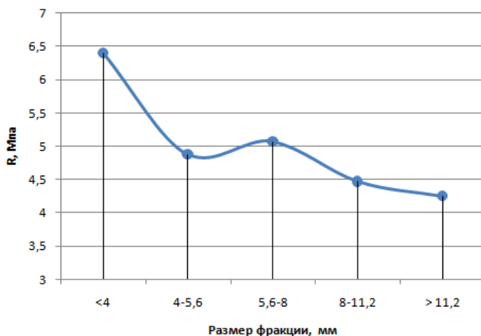
Рисунок 1 – Зависимость предела прочности асфальтобетона от размера фракции холодной гранулированной асфальтобетонной смеси
