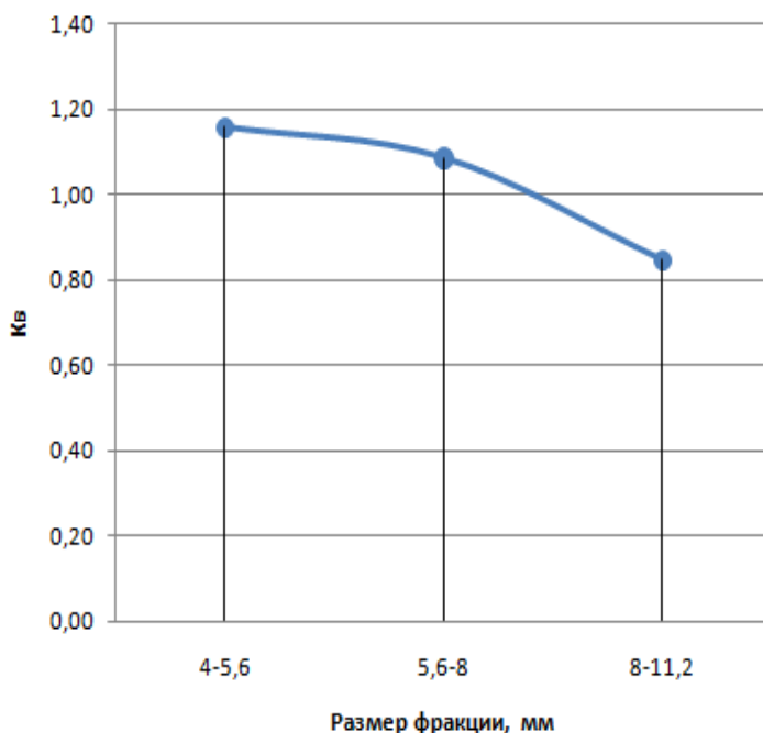
Рисунок 2– Зависимость коэффициента водостойкости асфальтобетона от размера фракции холодной гранулированной асфальтобетонной смеси
