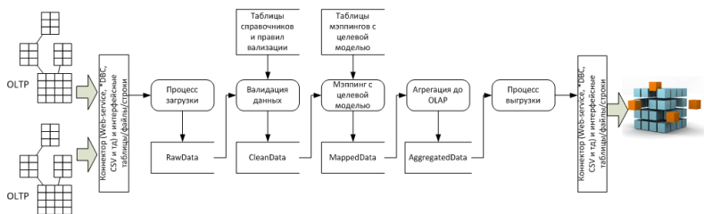
Рисунок 2 – Как работает ETL-система
