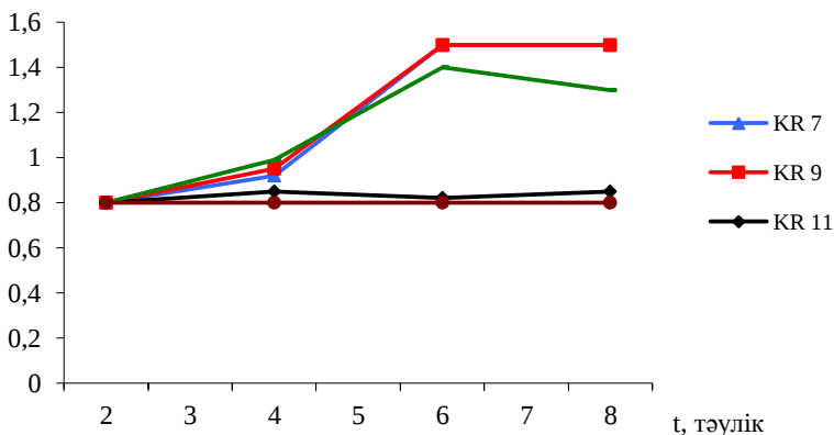
Сурет 2 – Дақылдардың мұнайы бар ортада өсу динамикасы
