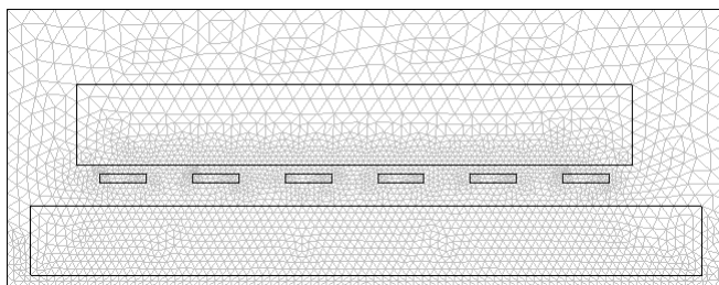
Рисунок 2 – Сетка конечных элементов
