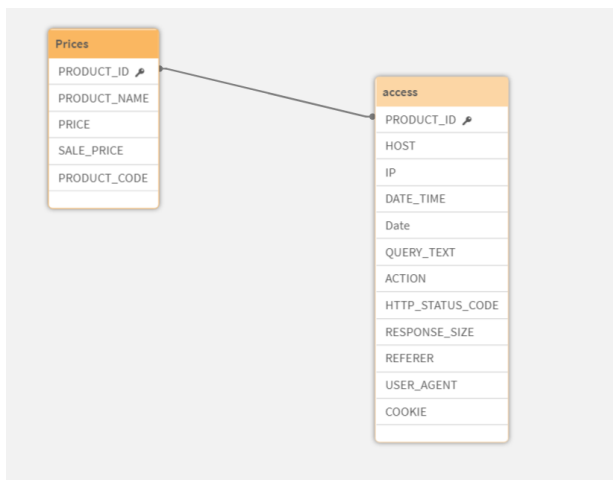
Рисунок 5 – Модель данных
