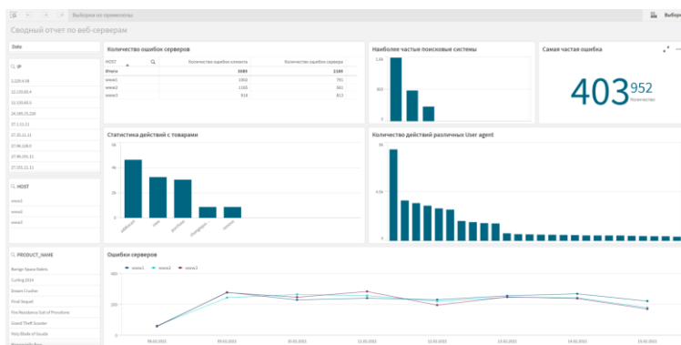
Рисунок 6 – Интерфейс приложения
