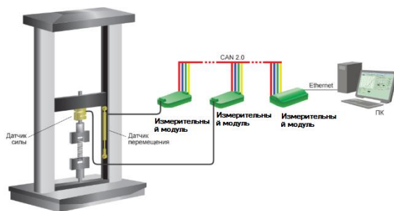
Рисунок 1 – Модель испытательной установки
