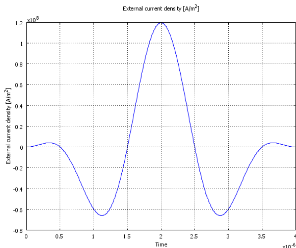
Рисунок 3 – Временная диаграмма плотности внешнего тока для ЭМАП
