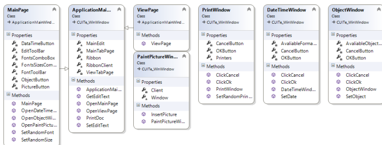
Рисунок 9 – Архитектура проекта UIFramework
