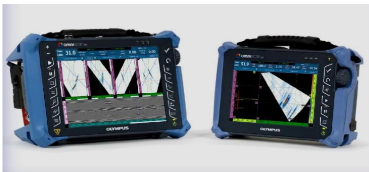
Рисунок 2 – Ультразвуковые дефектоскопы Olympus на фазированных решетках, МГц.
