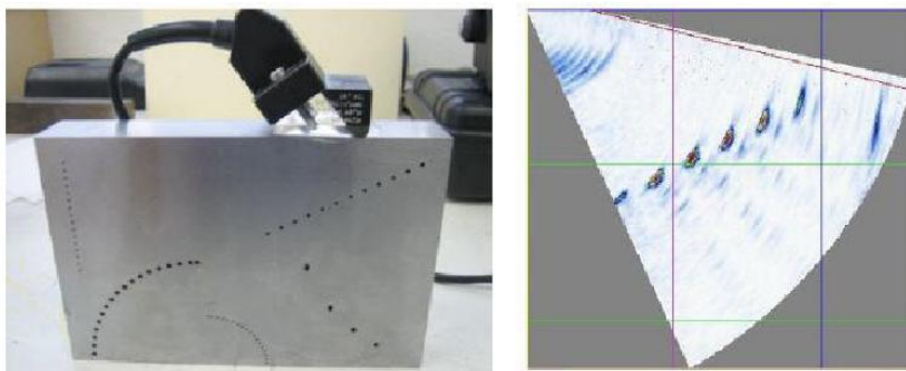
Рисунок 3 – Отображение дефектов на экране дефектоскопа на фазированных решетках
