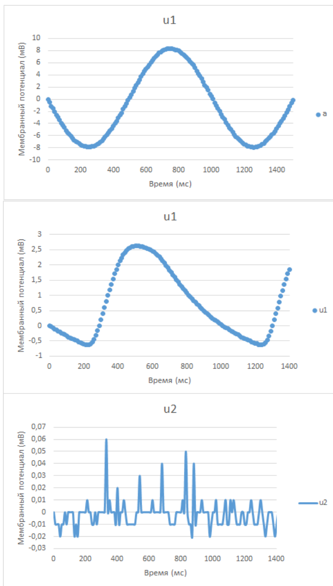
Рисунок 4 – A = 8B , S = \min , (а – входной сигнал, б – сигнал в теле нейрона, в – сигнал в аксоне)
