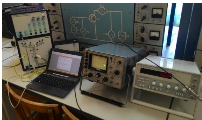
Рисунок 2 – Кобра 3: Нейросимулятор и генератор синусоидальных колебаний
