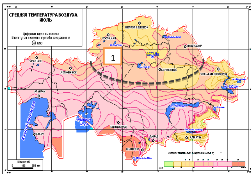
Рисунок 4 – Средняя температура воздуха в июле в Казахстане 1 – Ср. темп-ра воздуха в июле в Северном и Центральном Казахстане
