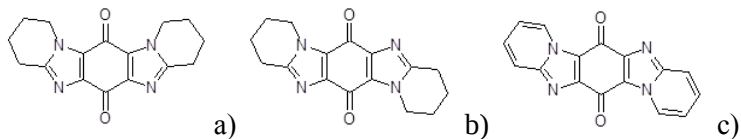
Рисунок 1 – Структуры а), б) противоопухолевых веществ, с) соединения, обладающего интенсивной флуоресценцией
