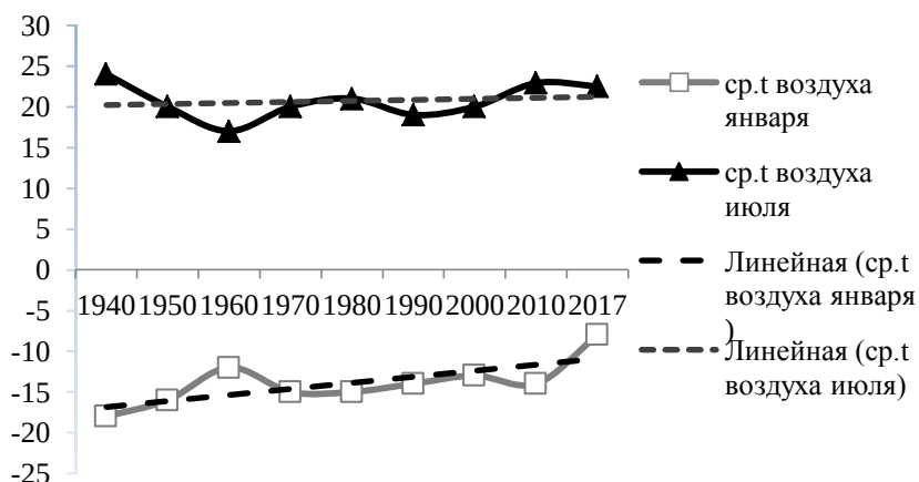
Рисунок 5 – Средняя температура воздуха в январе и в июле в г. Караганда за 1940–2017 гг.
