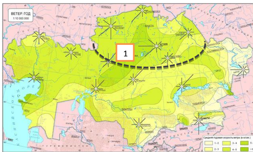
Рисунок 2 – Средняя годовая скорость и направление ветра в Казахстане
