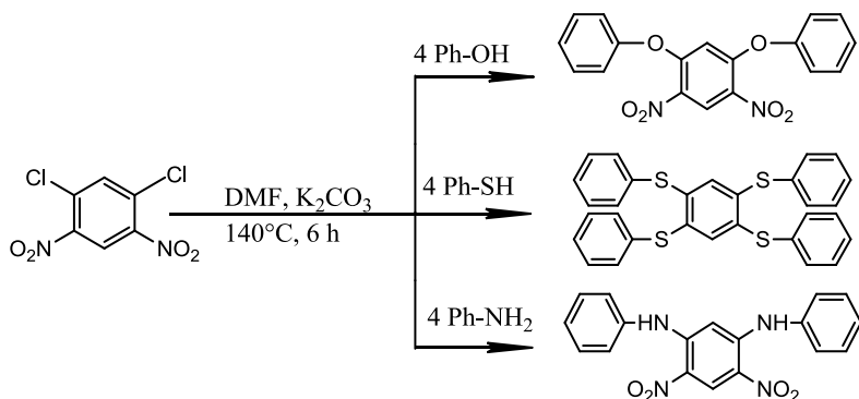
Рисунок 2 – Взаимодействие S-, O- и N-нуклеофилов с 1,5-дихлор-2,4-динитробензолом
