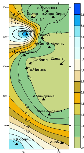
Рисунок 4 – Карта содержания тяжелых УВ в газах грязевых вулканов Бакинского архипелага
