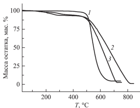
Рисунок 3 – Кривые термогравиметрический анализа ПФХ , полученных в растворе м -крезола (1), и в СК-CO 2 с использованием в качестве катализатора этилового спирта (2) и бензилового спирта (3)
