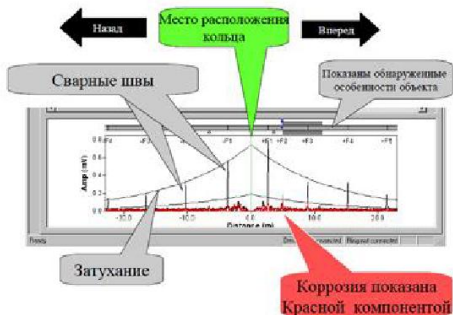
Рисунок 5 – Дефектограмма, полученная при обследовании трубопровода системой Wavemaker G4
