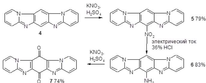
Схема 4 – Синтез 4a,5b,10,12-тетраазаиндено[2,1- b ]флуорен-5,11-диона
