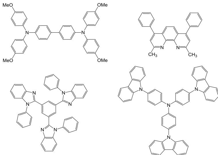
Рисунок 1 –Люминесцентные производные азотсодержащих гетероциклов
