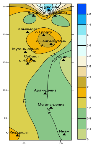
Рисунок 5 – Карта содержания углекислого газа в газах грязевых вулканов Бакинского архипелага
