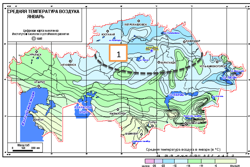
Рисунок 3 – Ср. темп-ра воздуха в январе в Казахстане
