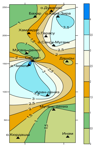
Рисунок 1 – Карта содержания азота в газах грязевых вулканов Бакинского архипелага
