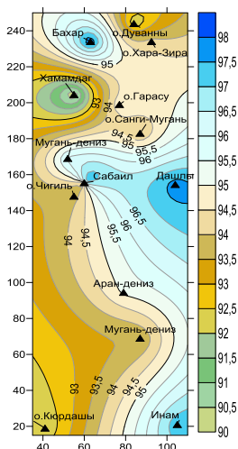
Рисунок 3 – Карта содержания метана в газах грязевых вулканов Бакинского архипелага
