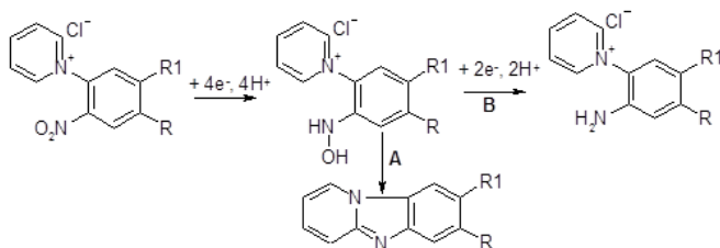
Схема 3 – Влияние свойств среды и температуры реакции на процесс восстановления дихлорида 1,1'-(4,6-динитро-1,3-фенилен)бис(пиридиния)
