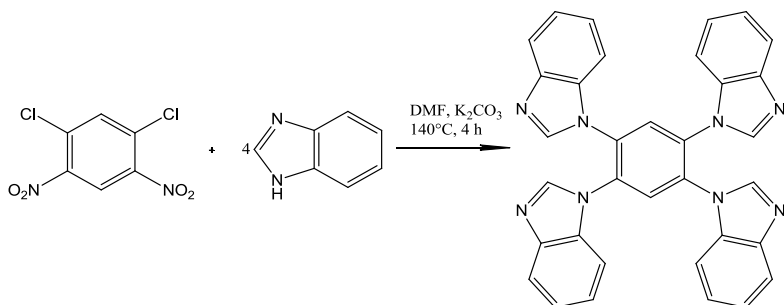
Рисунок 3 – Схема синтеза 1,2,4,5-тетракис(бензимидазолил)бензола
