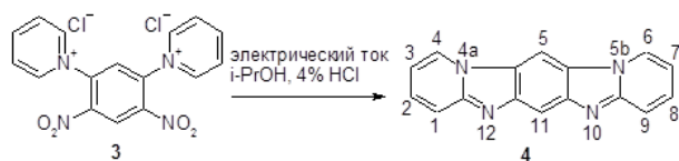
Схема 2 – Способ синтеза 4а,5b,10,12-тетраазаиндено[2,1- b ]флуорена (ТАИФ)
