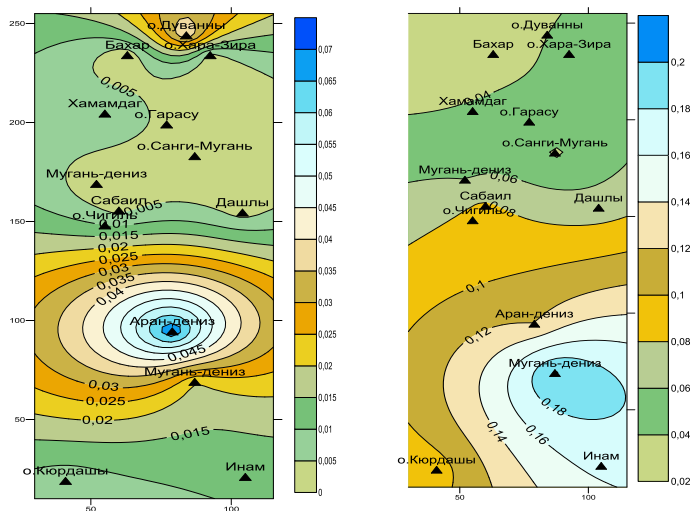
Рисунок 2 – Карта содержания гелия и аргона в газах грязевых вулканов Бакинского архипелага
