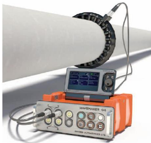
Рисунок 4 – Система комплексного сканирования трубопроводов Wavemaker G4
