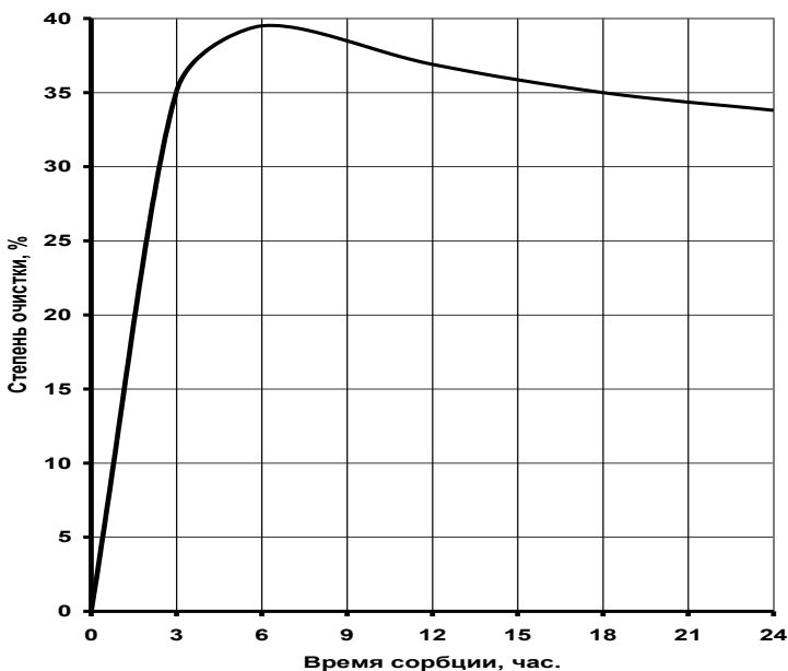
Рисунок 3 – Влияние времени контакта на степень очистки растворов от сульфат-иона при сорбции шунгитсодержащими алюмосиликатными сланцами
