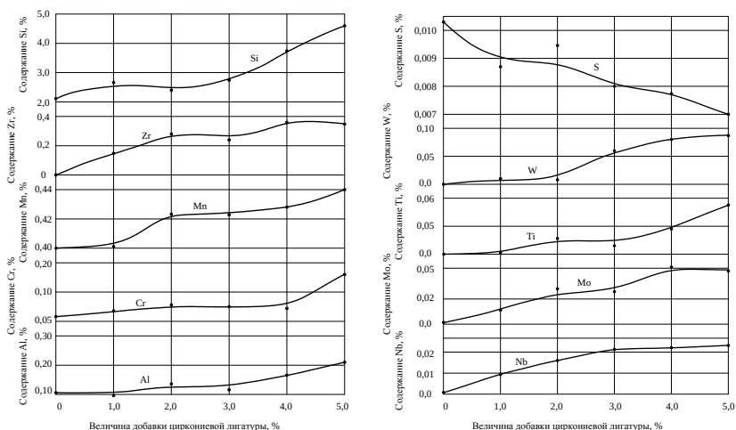
Рисунок 6 – Зависимость концентрации химических элементов в чугунах от величины добавки циркониевой лигатуры
