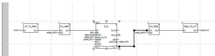
Рисунок 1 □ FBD-программа, реализующая регулирование расхода шихты на различные батареи аппаратов цеха по ПИД-закону
