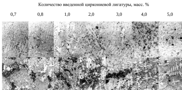
Рисунок 4 – Структура чугуна, охлажденного на установке «Параболоид» со скоростью 20 град/мин: x100: а – нетравленного; б – травленного
