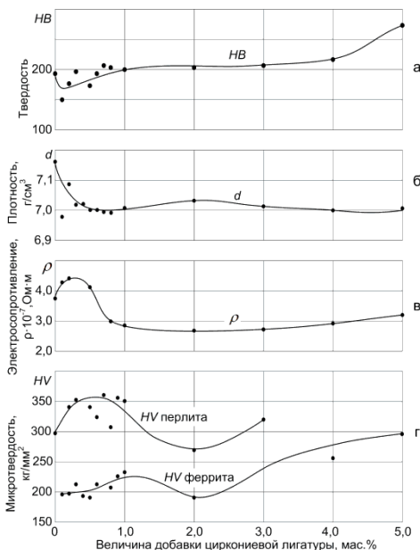
Рисунок 5 – Физико-механические свойства циркониевого чугуна
