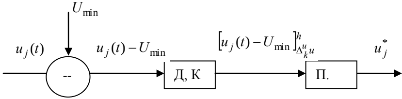
Рисунок 2 – Структурная схема АЦП
