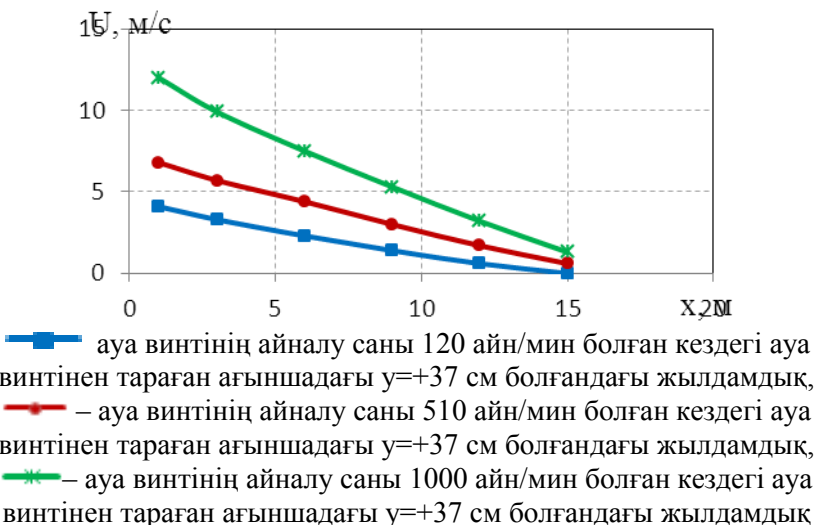
Сурет 1 – Ауа винтінің айналу саны 120 айн/мин, 510 айн/мин, 1000 айн/мин болған кездегі ауа винтінен тараған ағыншадағы U = f(x) \Rightarrow y = +37 см болғандағы жылдамдықтың винттен ара қашықтығына байланысты өзгеру графигі
