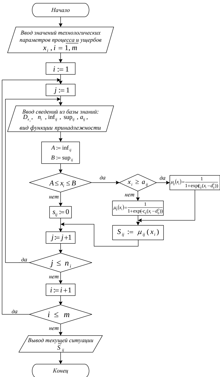
Рисунок – Алгоритм оценки текущей нечеткой ситуации
