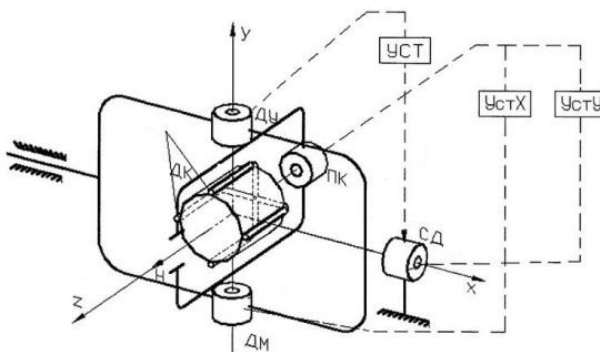
Рисунок 1 – Гиростабилизатор с перемещающимися массами
