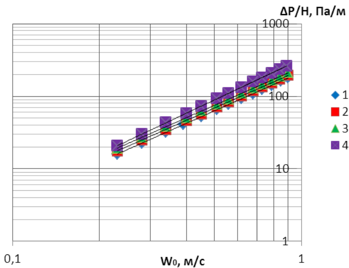
Рисунок 7 – Зависимость \Delta P/H = f(W_0) для сухой и орошаемой испытанной насадки: 1 – сухая насадка; 2 – орошение 4,8 \text{ м}^3/\text{м}^2\text{ч} ; 3 – орошение 9,6 \text{ м}^3/\text{м}^2\text{ч} ; 4 – орошение 14,3 \text{ м}^3/\text{м}^2\text{ч}
