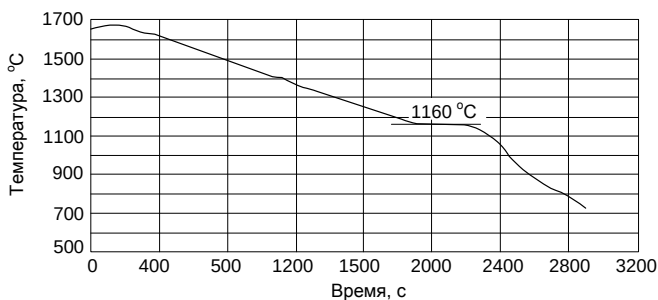
Рисунок 3 – График зависимости температура-время для циркониевой лигатуры
