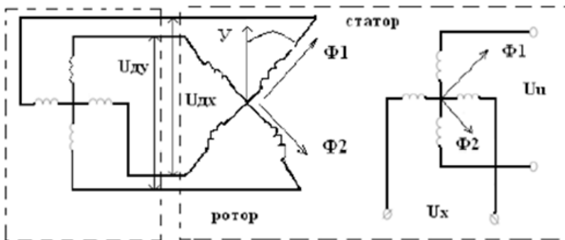
Рисунок 2 – Преобразователь координат
