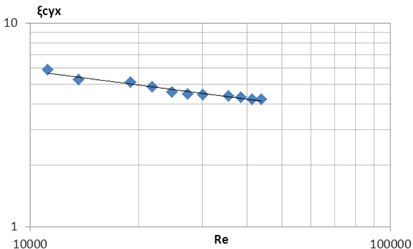
Рисунок 6 – Зависимость коэффициента сопротивления от числа Рейнольдса
