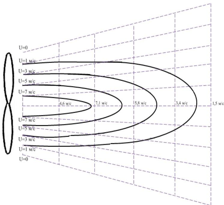
3 сурет – Ауа винтінің айналу саны 1000 айн/мин болған кездегі тараған ағыншадағы остік жылдамдықтың сұлбесі
