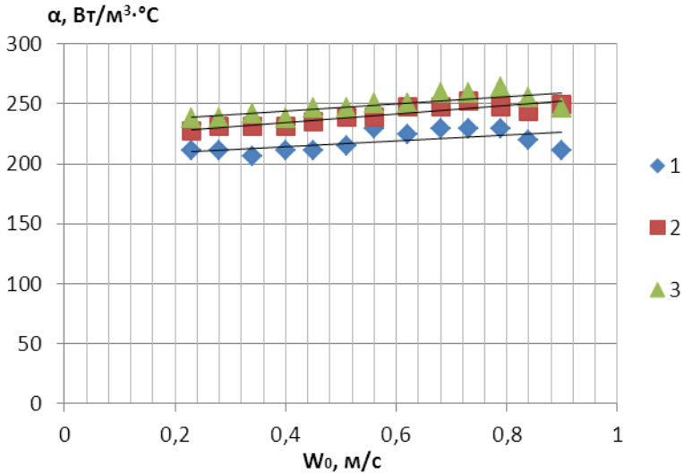
Рисунок 9 — Зависимость \alpha_v=f(W_0) : 1 — орошение 4,8 \text{ м}^3/\text{м}^2\text{ч} ; 2 — орошение 9,6 \text{ м}^3/\text{м}^2\text{ч} ; 3 — орошение 14,3 \text{ м}^3/\text{м}^2\text{ч}
