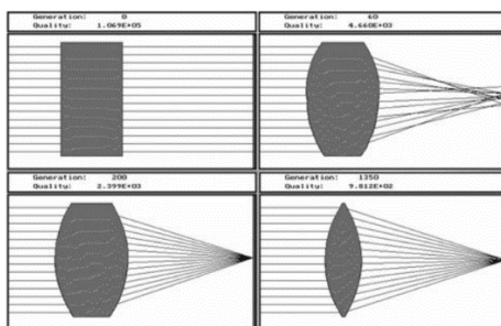
Рисунок 2 – Программа эволюционной оптимизации линзы Инго Рехенберга
