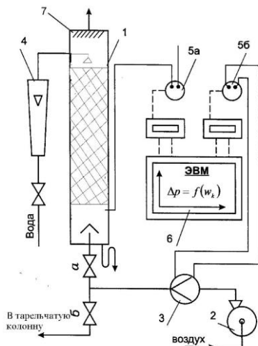
Рисунок 4 – Схема лабораторной установки: 1 – колонна; 2 – воздуходувка; 3 – измерительная диафрагма; 4 – ротаметр; 5 – манометры; 6 – ЭВМ; 7 – брызгоуловитель; а, б – регулировочные вентили
