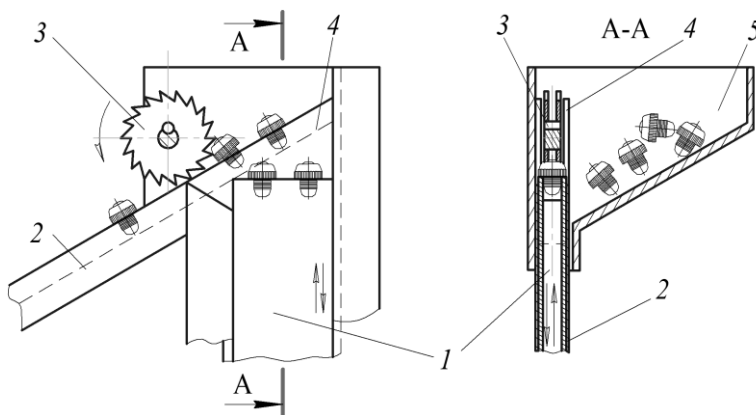
Рисунок 4 – Схема ножового бункерного загрузочного устройства: 1 – нож; 2 – лоток; 3 – сбрасыватель; 4 – приемник; 5 – бункер
