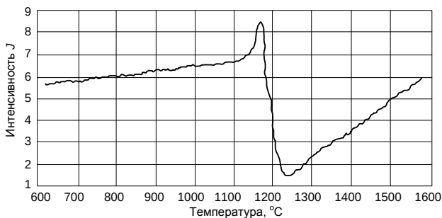
Рисунок 2 – Интенсивность \gamma -лучей, прошедших через циркониевую лигатуру в жидком состоянии в процессе охлаждения
