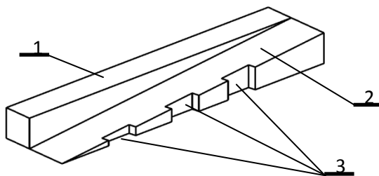
Рисунок 1 – Конструкция тест-фантома
