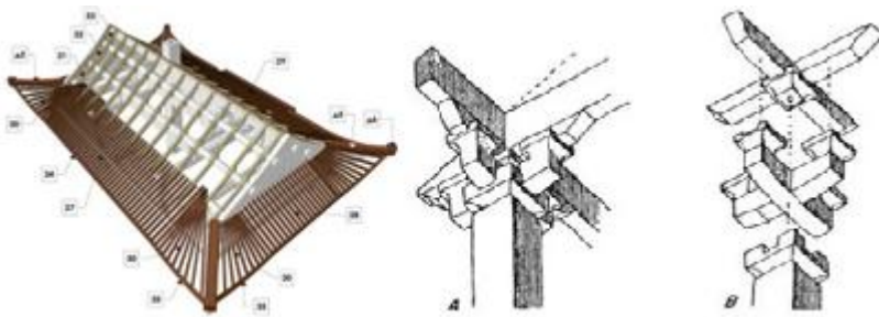
Рисунок 3 – Крыша в китайском стиле. Детали монументальной деревянной конструкции
