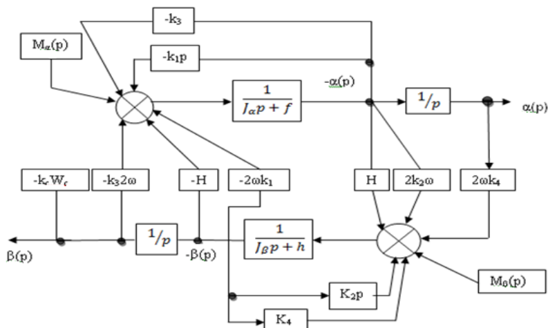
Рисунок 3 – Структурно-динамическая схема гиросtabilизатора
