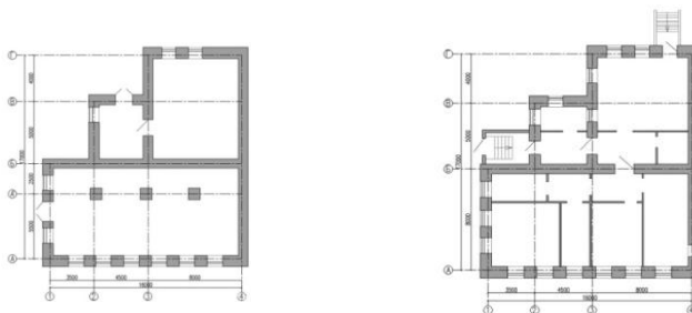
Рисунок 3 – План цокольного и 1-го этажа жилого дома, обмер 2016 г.
