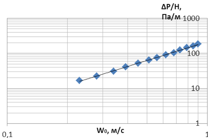
Рисунок 5 – Зависимость \Delta P/H = f(W_0) для сухой насадки из
