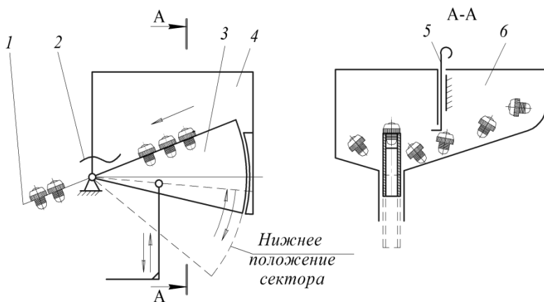
Рисунок 3 – Схема секторного бункерного загрузочного устройства: 1 – приемный лоток; 2 – сбрасыватель; 3 – сектор; 4 – бункер; 5 – заслонка; 6 – предбункер
