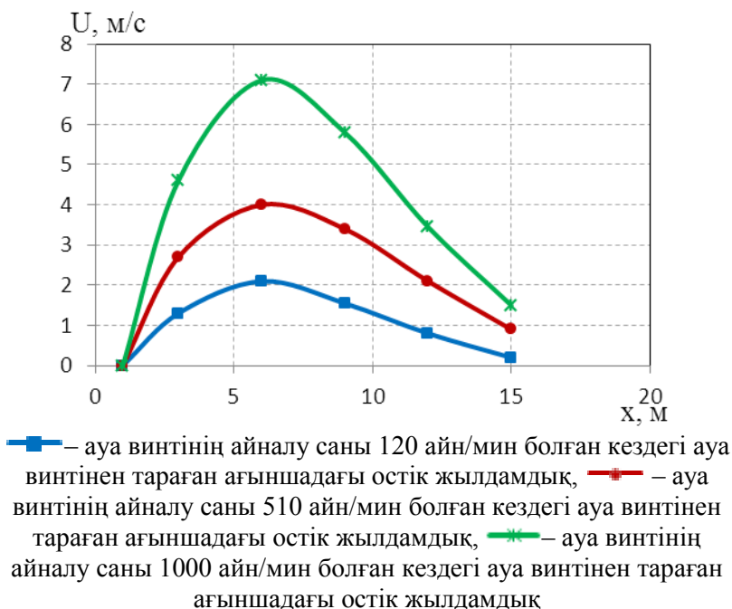
Сурет 2 – Ауа винтінің айналу саны 120 айн/мин, 510 айн/мин, 1000 айн/мин болған кездегі ауа винтінен тараған ағыншадағы остік жылдамдықтың винттен ара қашықтығына байланысты өзгеру графигі
