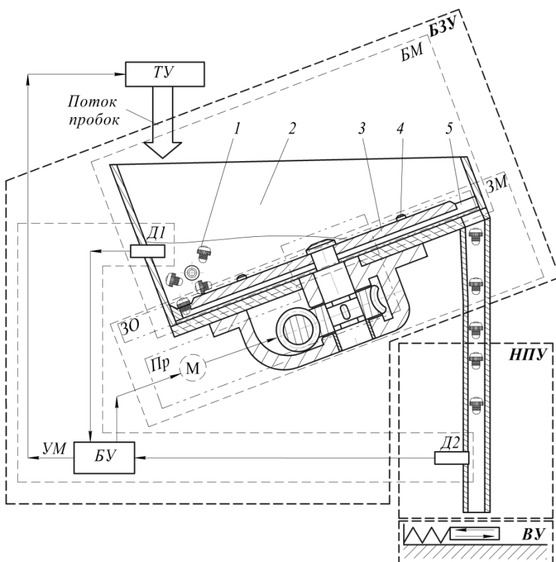
Рисунок 2 – Система автоматической загрузки Т-образных пробок в линии розлива алкогольных напитков
