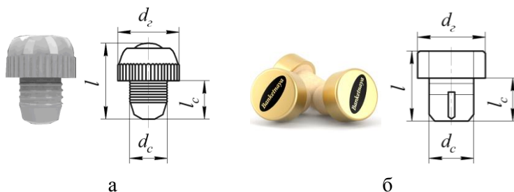
Рисунок 1 – Т-образные пробки для шампанского (а) и элитных алкогольных напитков (б)
