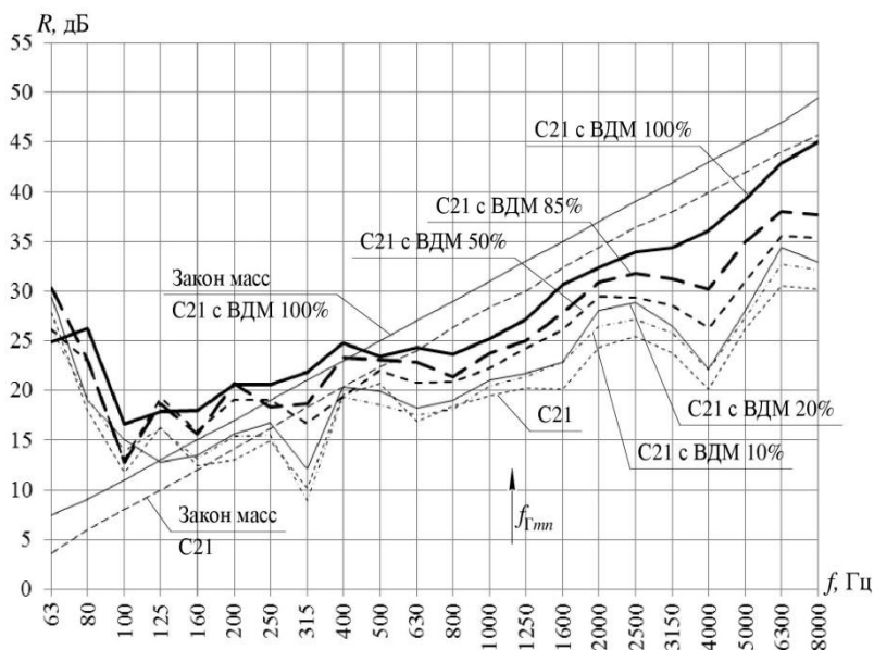
Рисунок 1 – Влияние коэффициента потерь на звукоизоляцию однослойной ортотропной пластины
