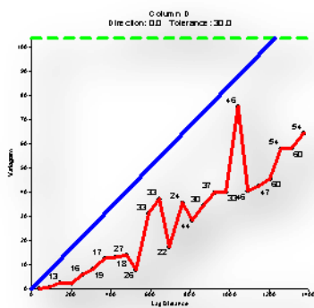
Рисунок 2 – вариограмма ( a ) и 3-D модель ( б ), построенные по данным о высотных отметках скважин
