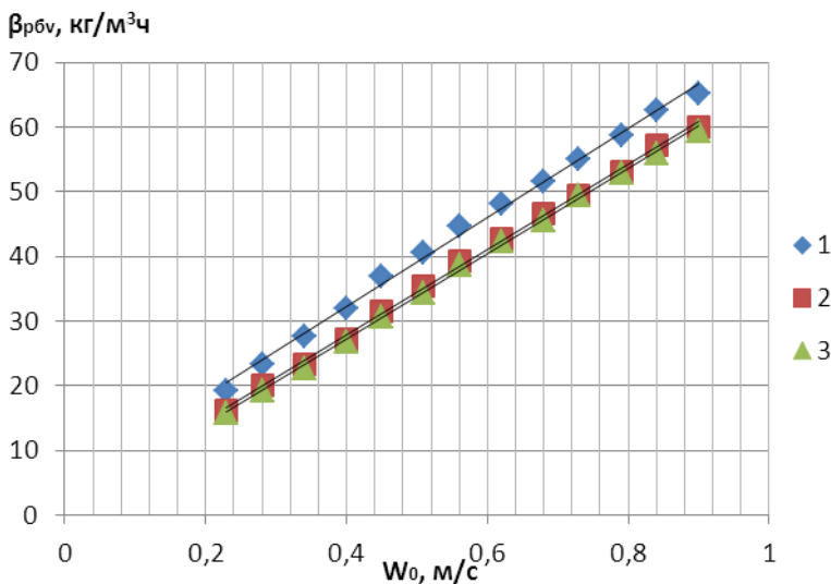
Рисунок 8 – Зависимость \beta_{p6v}=f(W_0) : 1 – орошение 4,8 \text{ м}^3/\text{м}^2\text{ч} ; 2 – орошение 9,6 \text{ м}^3/\text{м}^2\text{ч} ; 3 – орошение 14,3 \text{ м}^3/\text{м}^2\text{ч}
