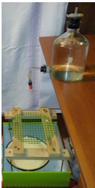
Рисунок 2 – Установка для изучения особенностей растекания одиночной струи капельной жидкости по поверхности насадки
