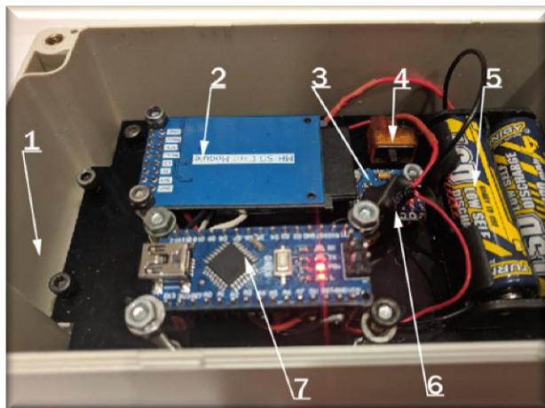
Рисунок 1 – Общий вид экспериментального прибора для пространственного позиционирования трубопровода. 1 – влагозащищенный корпус; 2 – кардридер; 3 – сенсор (гироскоп+акселерометр); 4 – выключатель; 5 – источник питания; 6 – преобразователь напряжения; 7 – микроконтроллер.
