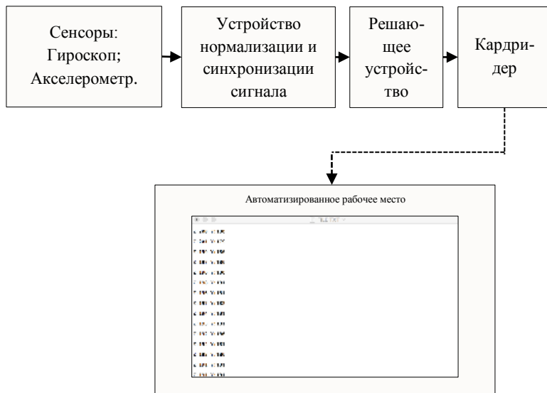
Рисунок 2 – Блок-схема прибора
