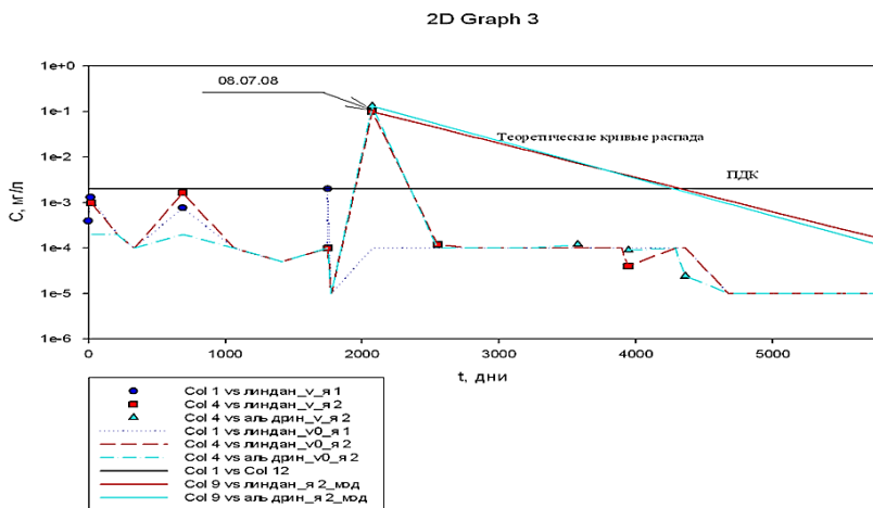
Рисунок 4 – Концентрации линдана и альдрина в шахтах Я1 и Я2. Для удобства ось ординат дана в логарифмическом масштабе. Теоретические кривые проведены по уравнению (3) с использованием параметров, приведенных в таблице 2
