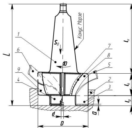
Рисунок 1 – Резцовая головка
