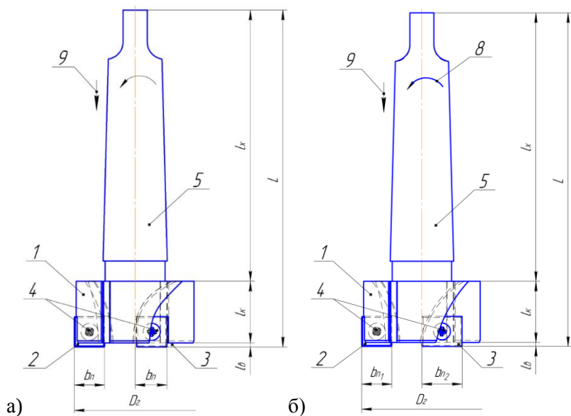
Рисунок 2 – Сборная резцовая головка с твёрдосплавными пластинами одинаковой (а) и разной (б) ширины
