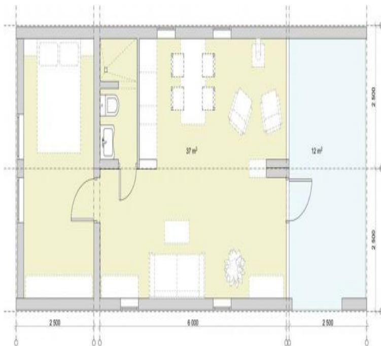
Рисунок 1 – Типовой план «Дубль Дом»
