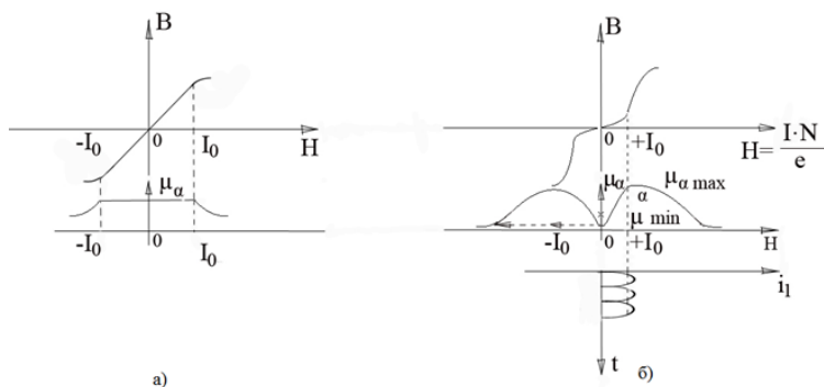
Рисунок 2 – Кривые намагничивания.
