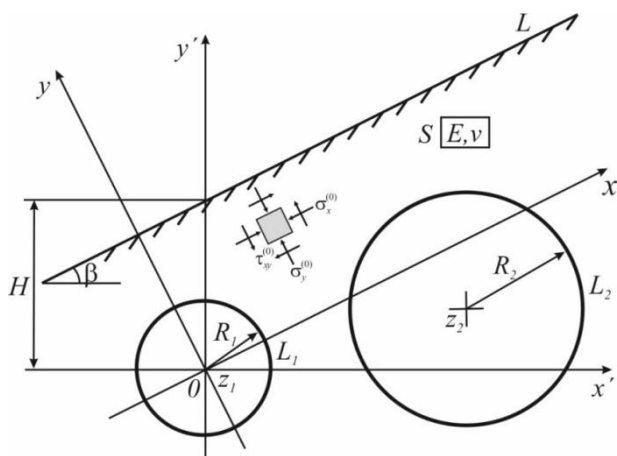
Рисунок 1 – Расчетная схема
