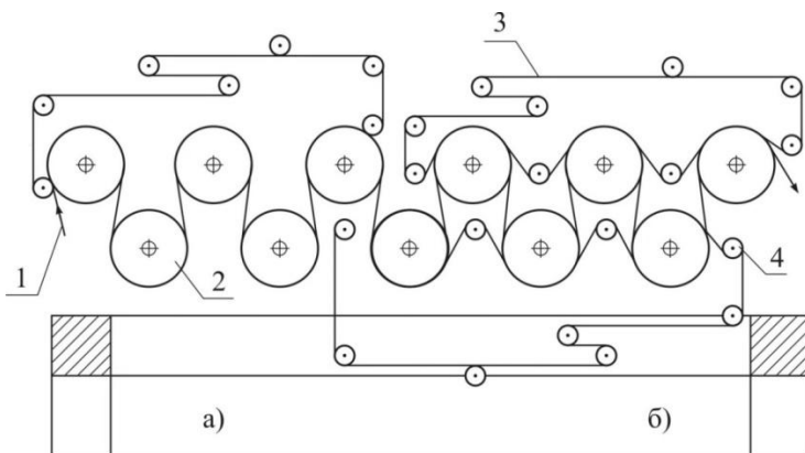
Рисунок 1 – Схема проводки бумажного полотна в сушильной части бумагоделательной машины: а) – безобрывная проводка; б) – традиционная проводка; 1 – бумажное полотно; 2 – сушильный цилиндр; 3 – сушильная сетка; 4 – направляющий вал
