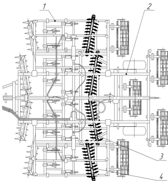
Рисунок 1 - Схема агрегата
