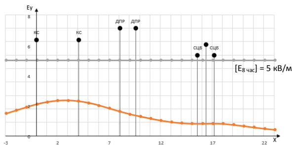
Рисунок 3 – Блок вывода результатов расчета напряженности электрического поля
