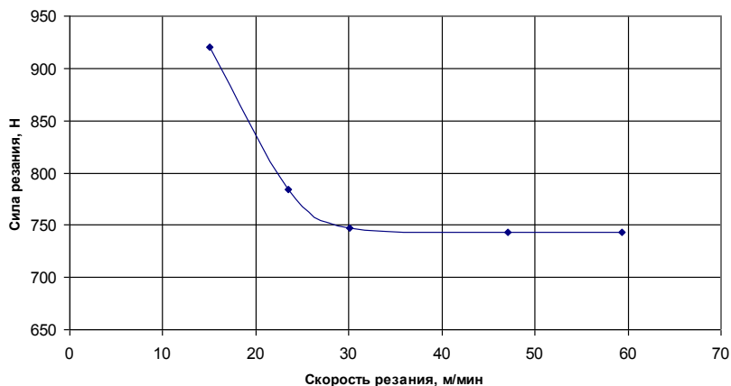
Рисунок 3 – Зависимость силы резания от скорости резания при обработке титанового сплава ВТ6 (глубина резания t = 1,5 мм; подача S_o = 0,15 мм/об).
