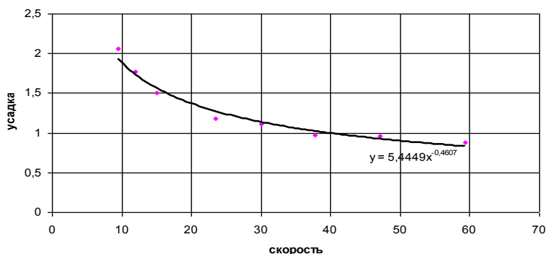
Рисунок 4 – Зависимость коэффициента поперечной усадки стружки от скорости резания при обработке титанового сплава ВТ6 (глубина резания t = 1,5 мм; подача S_o = 0,15 мм/об)
